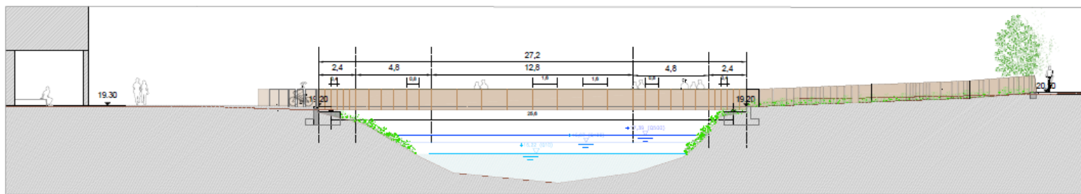
ALZADO SUR
